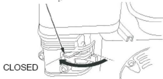
Важіль повітряної заслінки
